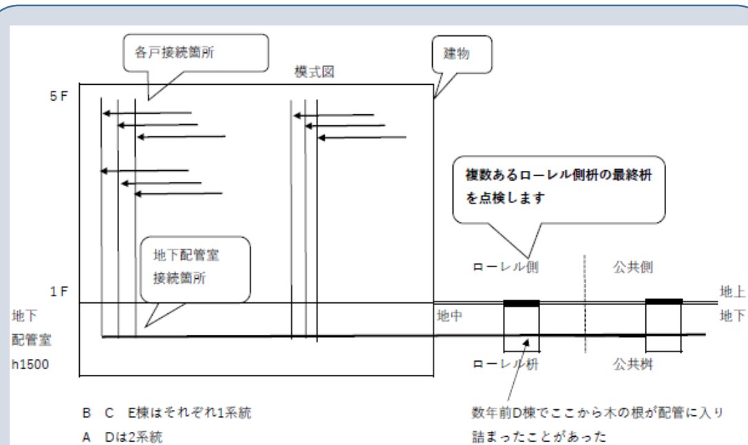
▲トイレの使用可否を判断する際の排水配管の確認箇所図
